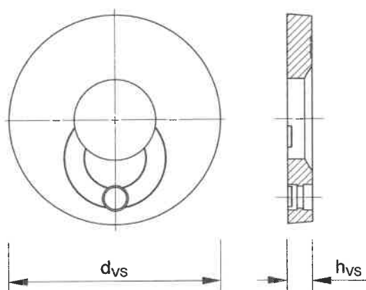
Podkładka uszczelniająca
